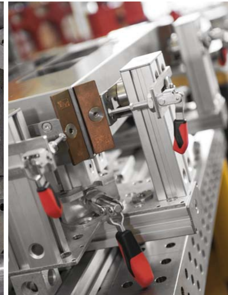
> Baukastensystem für Vorrichtungen zum automatisierten Schweißen > Construction kit system for automated welding fixtures
