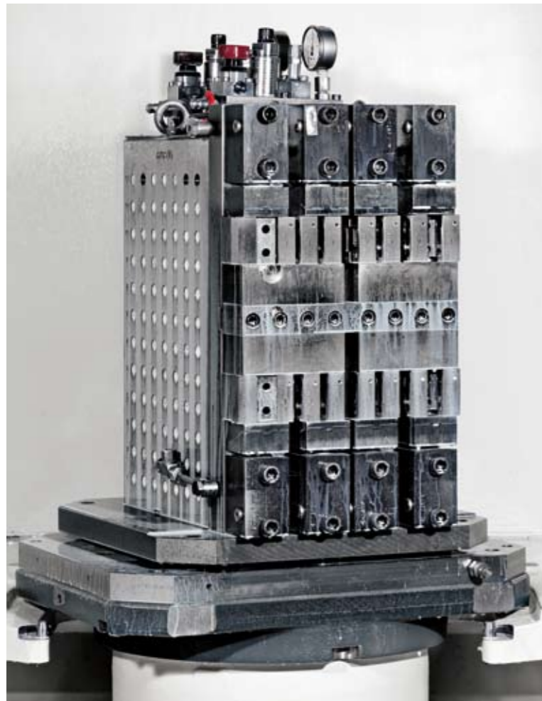
> Systemlösung aus modularer, hydraulischer und Nullpunkt-Spanntechnik > System solution featuring modular, hydraulic and zero point clamping technology
