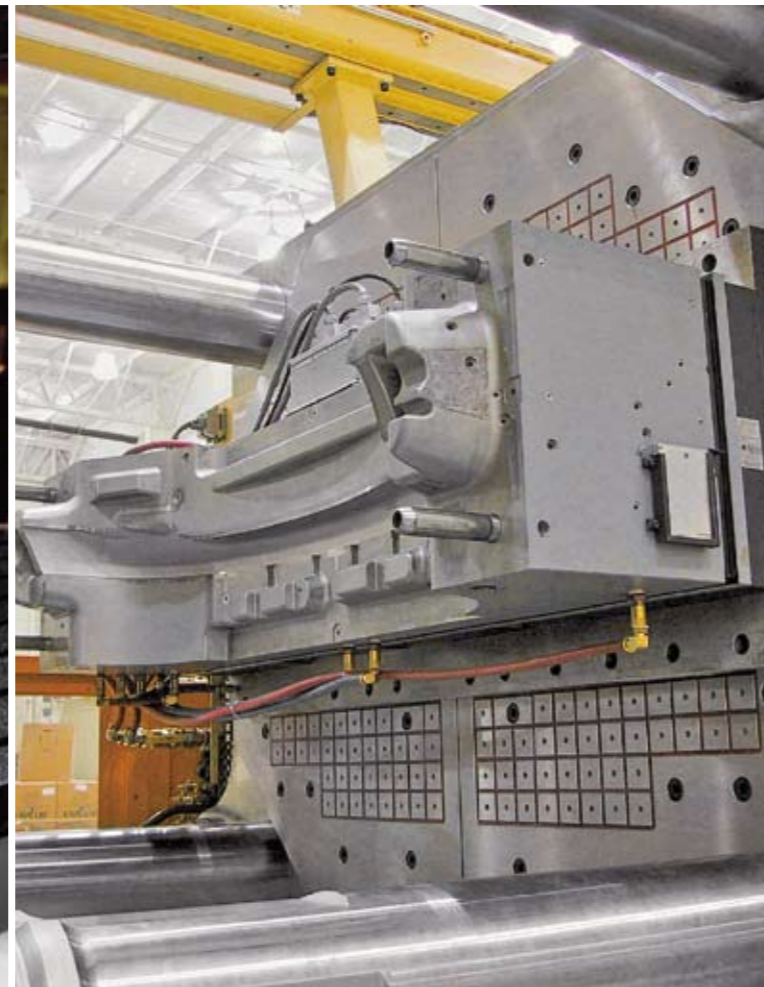
> Hohe Haltekräfte durch die AMF-Magnetspanntechnik auch beim Spritzgießen > High retaining forces courtesy of AMF magnetic clamping technology, including for injection moulding
