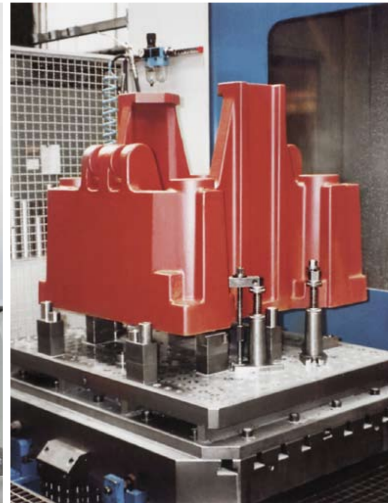
> Modulare Spanntechnik für die Großteilefertigung > Modular clamping technology for manufacturing large parts
